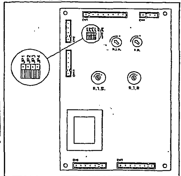
STEUERPLATINE
