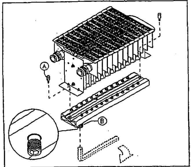
BRENNEREXPLOSIONSZEICHNUNG
